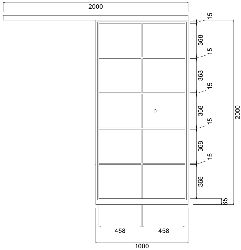
1-flügelige Stahl Schiebetür
